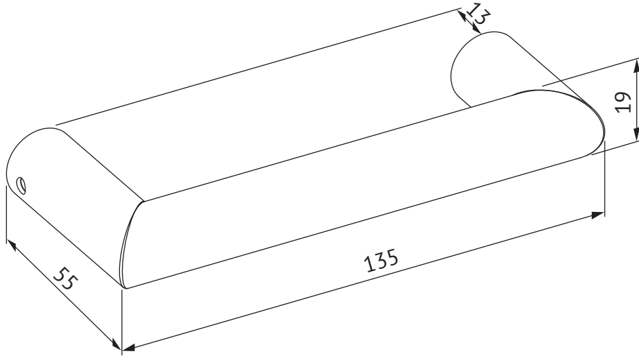
Scandinavian / DIN LH002
